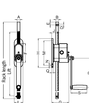
Model ZWW-L, nosnosť 250 - 500 kg
