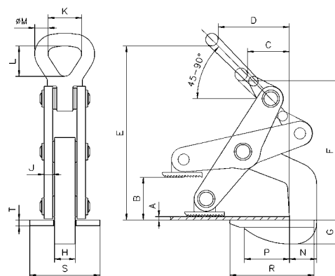
Model TWH s doštičkou
