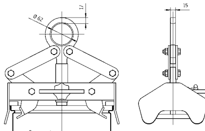
Model TKA.../...i s vnútorným úchopom
