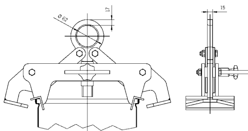
Model TKA.../...s vonkajším úchopom
